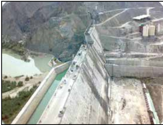
نگاره ۱۶- نمایی از سد بتن غلتکی زبردان- چابهار (از اینترنت)
