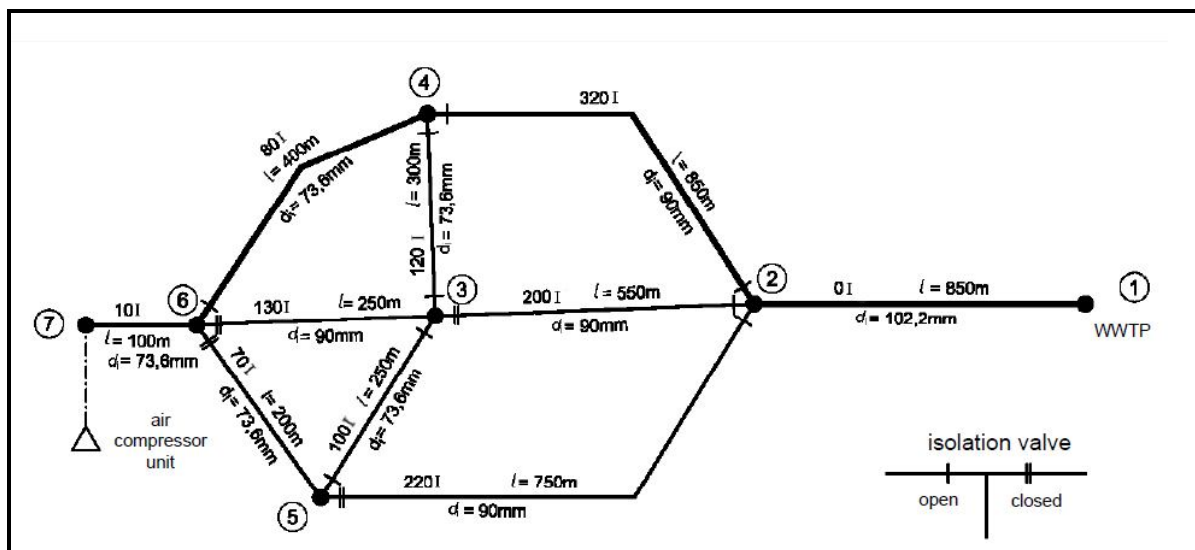
شکل پ.۱-۱- دیگران شماتیک مثال تعیین مشخصات تلمبه و قطر لوله
