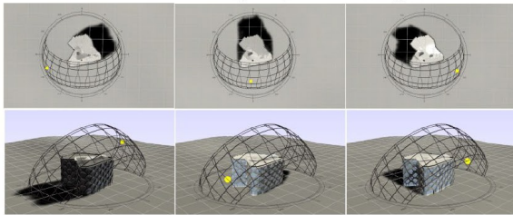
مطالعه تابش در ساعات و فصول مختلف
